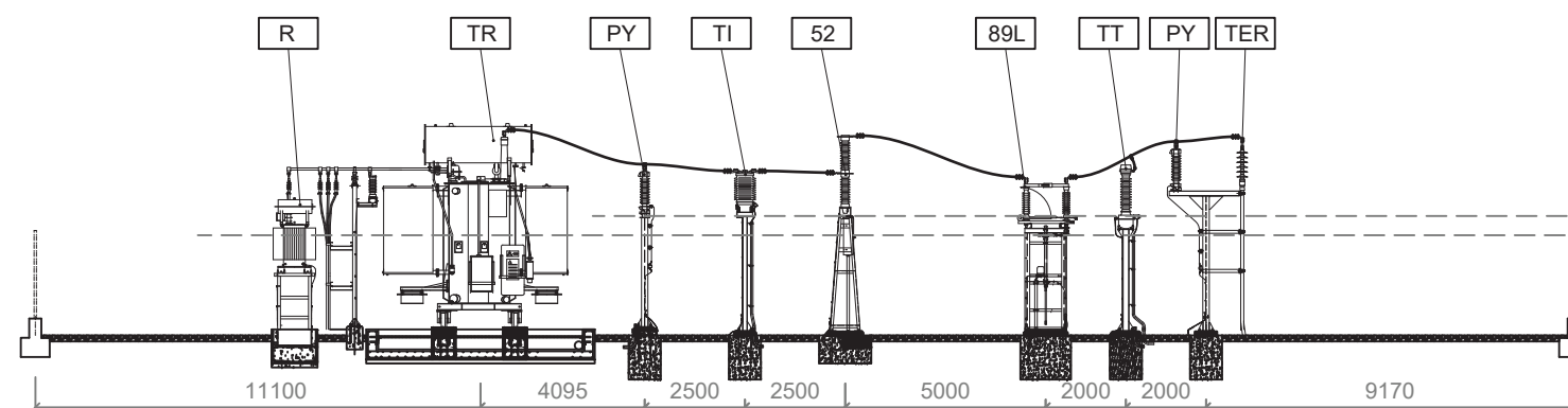
SECCIÓN A-A
